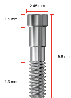
Zentralschraube Central Screw
