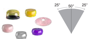
Prothetik-Set (Smart box) Prosthetic Set (Smart box) Art.-Nr / Item-No: 335SBC Divergenzausgleich bis max. 50° Divergence compensation up to max. 50°
