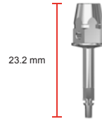
Universaleindrehhilfe (Kurz)* Universal Insertion Tool (Short)* (für Drehmomentratsche / for torque ratchet) Art.-Nr / Item No: 140331tra
