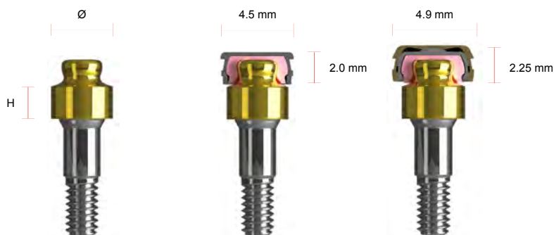
OT Equator® OT Equator® OT Equator® mit INOX Gehäuse OT Equator® with INOX housing OT Equator® mit Smart Box OT Equator® with Smart Box
